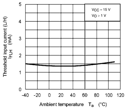
Fig. 13.2.4 I_{FLH} - T_a
