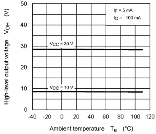
Fig. 13.2.8 V_{OH} - T_a
