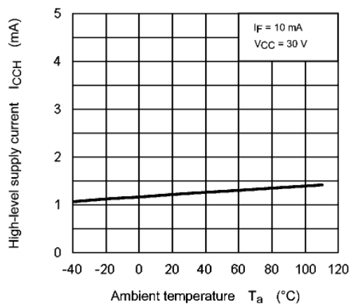
Fig. 13.2.6 I_{CCH} - T_a
