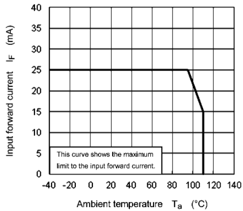
Fig. 13.2.2 I_F - T_a
