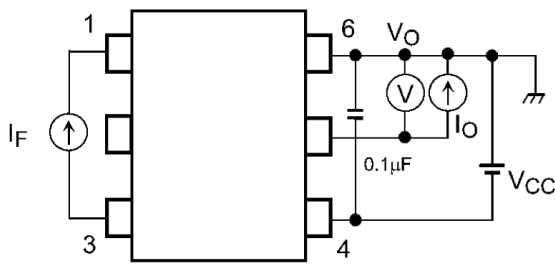
Fig. 13.1.1 I OPH Test Circuit
