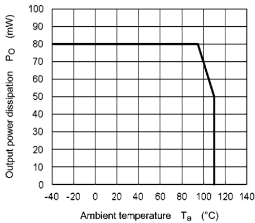
Fig. 13.2.3 P_O - T_a
