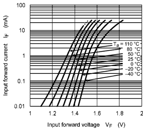
Fig. 13.2.1 I_F - V_F
