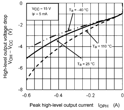
Fig. 13.2.10 (V_{OH} - V_{CC}) - I_{OPH}
